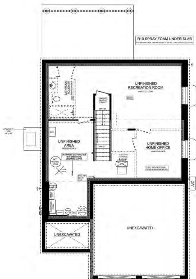
OAKMONT 'A' BASEMENT PLAN
