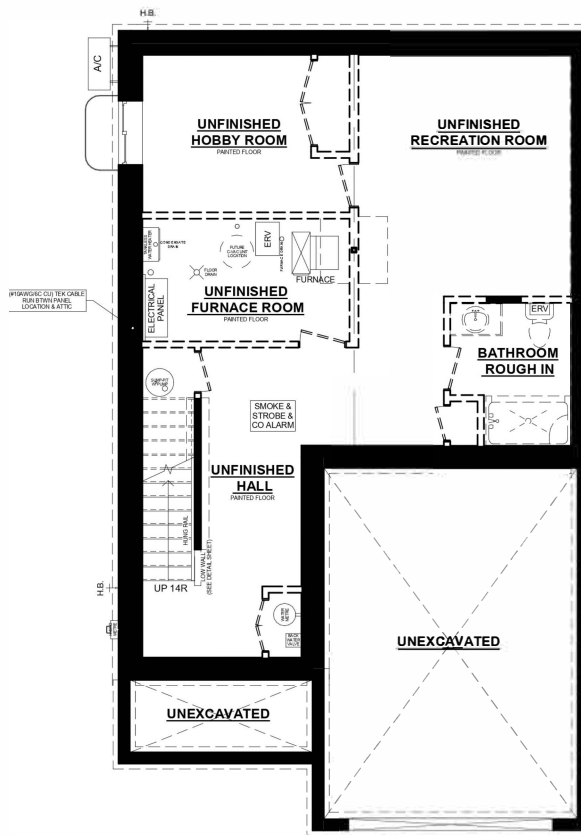
SEDONA 'B' UNIT #1 BASEMENT PLAN
