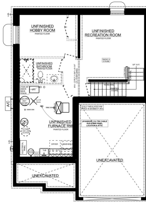
ELMWOOD 'B' UNIT #1 BASEMENT PLAN
